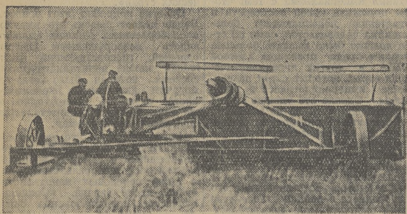
Общий вид переоборудованной лафетной жатки.
