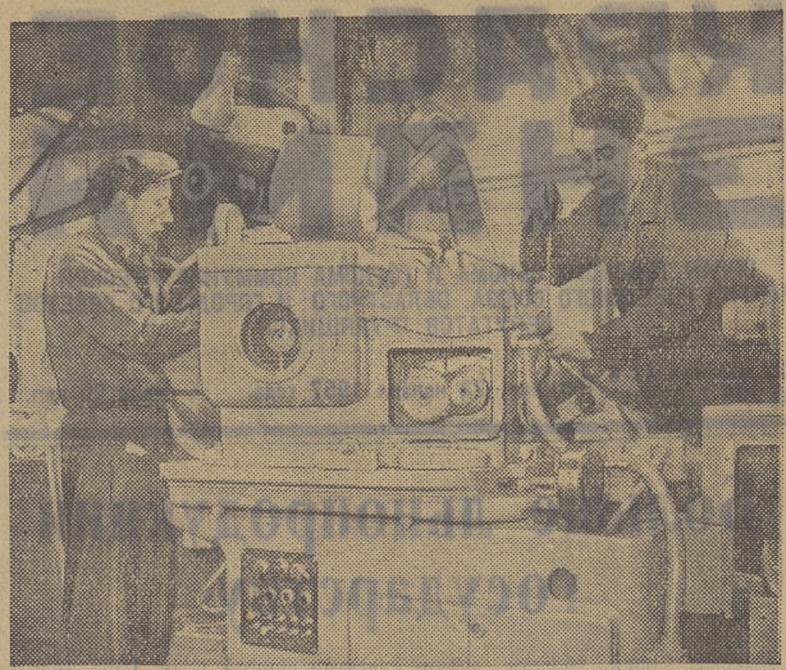
МОСКВА. На заводе внутришлифовальных станков изготовлен бесцентрово-шлифовальный автомат для автоматической линии 1-го подшипникового завода. Автомат производит шлифовку беговой дорожки внутреннего кольца роликового подшипника. На снимке: слесарь-сборщик Е. С. Малишев (слева) и электрик В. Н. Петрикин проводят окончательную отладку станка. (Фотохроника ТАСС).
