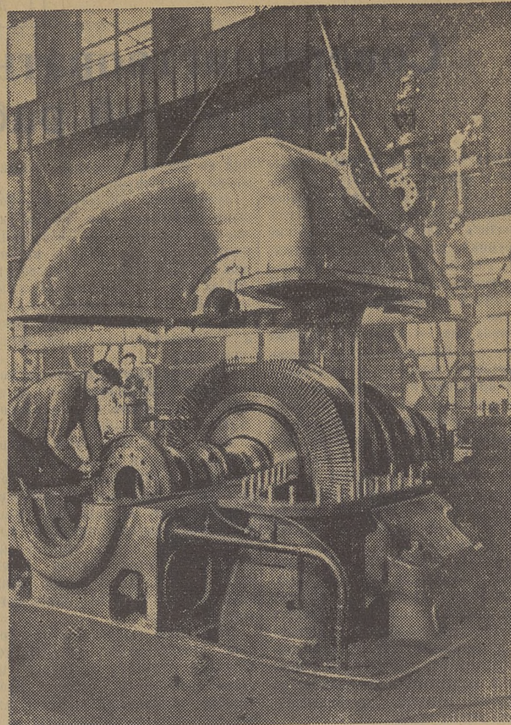
Брянский машиностроительный завод. На снимке: сборка турбины мощностью 12 тысяч киловатт, изготовляемой по заказу для Индии. (Фотохроника ТАСС).
