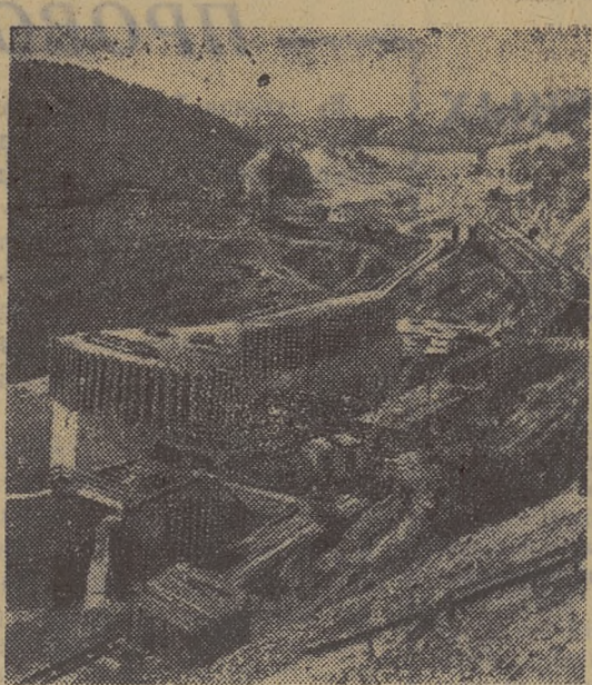
Народная Республика Болгария. На реке Тополница строится большое водохранилище. Высота плотинного водохранилища достигает 78 метров, а длина — 326 метров. Размер водохранилища: длина составляет примерно 12 километров, ширина в ряде мест — 3 километра. Оно будет вмещать 140.000.000 кубометров воды. Будущее водохранилище даст возможность приводить в движение турбины электростанции, орошать 400.000 декар земли (декар — 1/10 гектара) в Пловдивской и Пазарджикской областях. На снимке: сооружение плотинного водохранилища «Тополница». (Фотохроника ТАСС).
