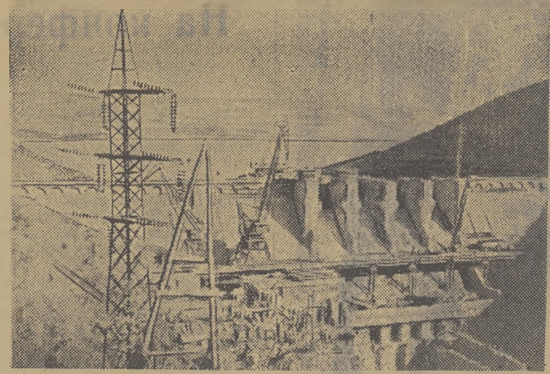
В Народной Республике Албания подходят к концу работы по строительству водосливных сооружений гидроэлектростанции имени Энвера Ходжи на реке Мати. В середине будущего года электростанция войдет в строй действующих предприятий. После окончания строительства мощность станции достигнет 20.000 киловатт.
