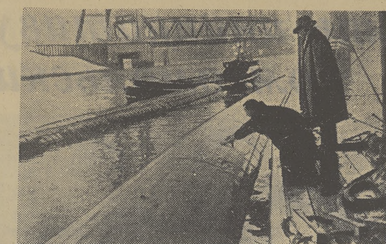
В Гамбурге (Федеративная Республика Германия) недавно демонстрировалось изобретение инженера Эрнста Дёрпнихауса — трубы из пластмассы для перевозки нефти. Они сделаны из очень дешевого материала, что является их преимуществом. Трубы, наполненные нефтью, могут быть погружены в воду на глубину около трех метров и прикреплены к буксиру, который доставит их к месту назначения. К одному буксиру можно прикрепить до четырех труб. На снимке: трубы из пластмассы для перевозки нефти в Гамбургском порту. (Фото агентства Рейстон).
