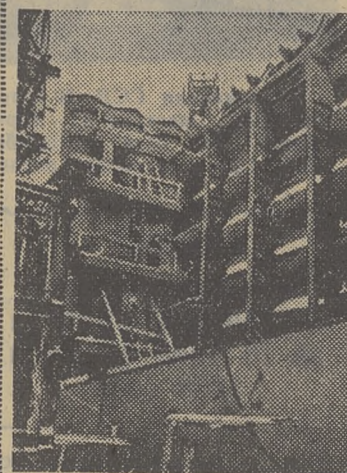
ЛЕНИНГРАД. Судостроители Балтийского завода имени С. Орджоникидзе работают над созданием танкера водоизмещением около 40 тысяч тонн. Такое крупное судно в Советском Союзе строится впервые.
