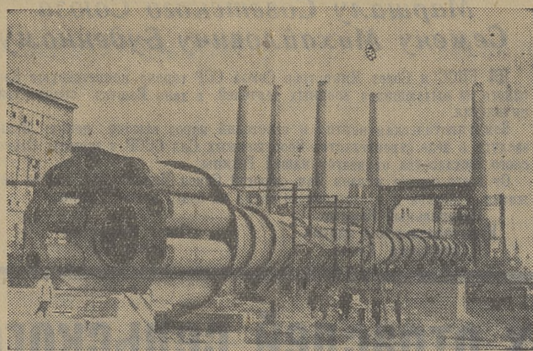
Белгородский цементный завод — один из крупнейших в стране. Он выпускает цемент высоких марок. Сейчас здесь монтируется первая вращающаяся 150-метровая печь. Пуск ее намечается к 1 мая.
