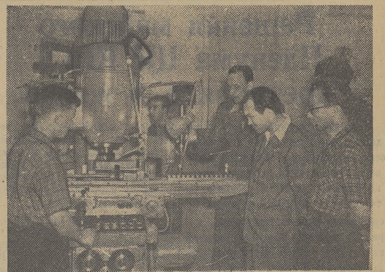
На снимке: в павильоне «Станкостроение». Наладчик Дмитрия Кузнецова фрезерных станков А. Кудряшов демонстрирует посетителям продукцию своего завода — вертикальный консольно-фрезерный копиральный станок с программным управлением (модель 6Н11КГ).
