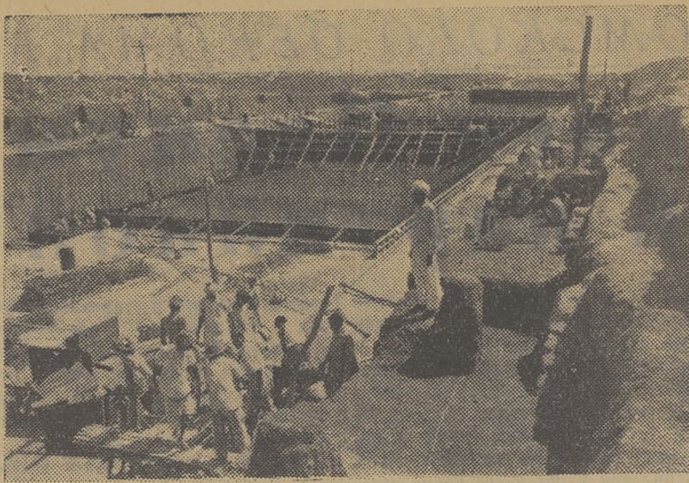
Индия. На строительстве металлургического комбината в Бхилиан. На снимке: на участке строительства прокатного цеха. (Фотохроника ТАСС).
