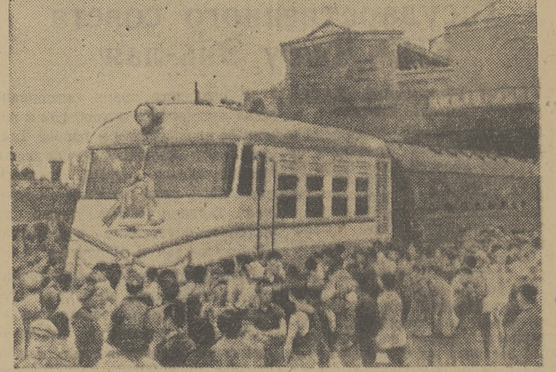
Китайская Народная Республика. Паровозостроители Чансинь-дунского завода (близ Пекина) в честь приближающейся девятой годовщины образования КНР построили первый отечественный тепловоз. Все его оборудование создано на заводах Китая. Новый локомотив снабжен дизелем мощностью 600 лошадиных сил и может развивать скорость до 85 километров в час.
