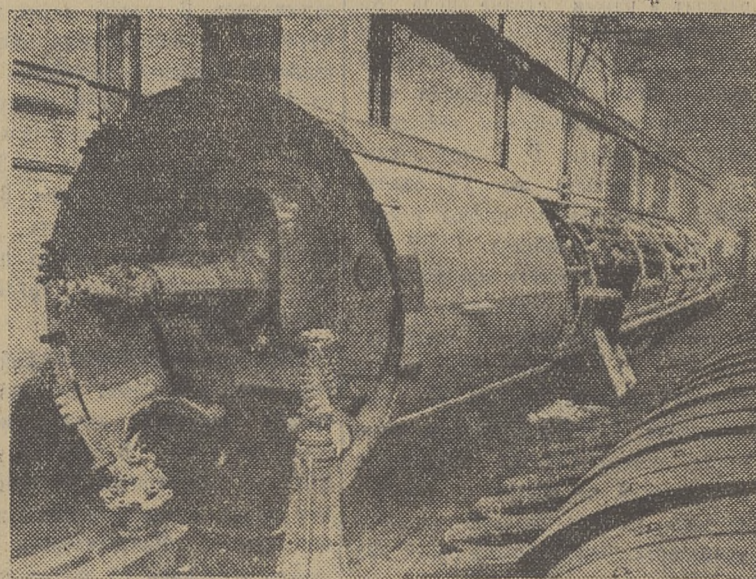
Тулеская область. На Узловском машиностроительном заводе изготовлен проходческий щит ПШМ-4. Он предназначен для прохождения горизонтальных горных выработок в сложных гидрогеологических условиях Подомосковского бассейна. Благодаря этому щиту полностью механизированы проходческие работы: разрушение породы и угольного пласта в забое, уборка и погрузка угля в вагонетки, возведение постоянной железобетонной крепи, все вспомогательные проходческие операции. Проектная скорость прохождения двухпутевой выработки — 330 погонных метров в месяц. На снимке: проходческий щит.
