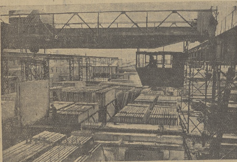
МОСКВА. На заводе железобетонных изделий № 12 освоено изготовление панелей, перегородок и внутренних стен на новых касетноформовочных машинах. Новая касетноформовочная машина разработана и внедрена работниками Карачаровского механического завода совместно с рабочими и инженерно-техническими работниками завода железобетонных изделий № 12. На снимке: общий вид склада готовой продукции, изготовленной касетным способом. (Фотохроника ТАСС).
