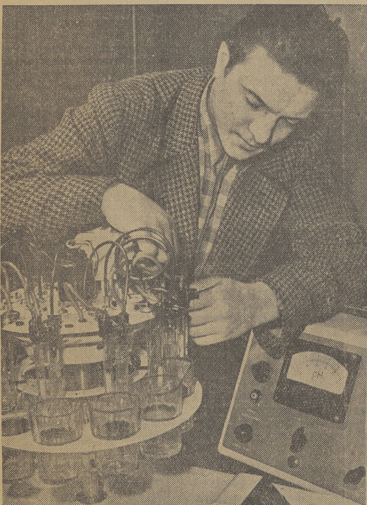
Существующий способ определения кислотности или щелочности почв трудоемок и требует больших затрат времени. Большой интерес поэтому представляет новый прибор, разработанный сотрудниками Центрального конструкторского бюро пищевого машиностроения и приборостроения. Он дает возможность производить быстрый массовый лабораторный контроль кислотности почв.
