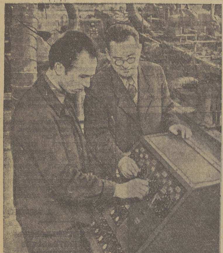
КИЕВ. В Украинском научно-исследовательском институте механической обработки древесины группа научных сотрудников под руководством кандидата технических наук Г. Н. Косовского создала первую в СССР автоматическую линию с программным управлением. На этой универсальной линии можно обрабатывать различных размеров бруски, детали мебели и стальных изделий. Система программного управления позволяет быстро перенастраивать работу станка. Время их настройки сокращается в 15—20 раз по сравнению с существующими автоматическими линиями. На снимке: старший техник лаборатории автоматики М. П. Стрижевский (слева) и кандидат технических наук Г. Н. Косовский у пульта управления новой автоматической линии. (Фотохроника ТАСС).
