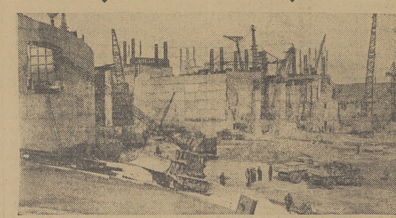
ВОЛЖСКИЙ. Строители Сталинградского ГЭС заканчивают сооружение судоподъемных шлюзов. С открытием навигации волжские корабли пойдут через шлюзы по новому руслу Волги. На снимке: общий вид строительства судоподъемных шлюзов. (Фотохроника ТАСС).
