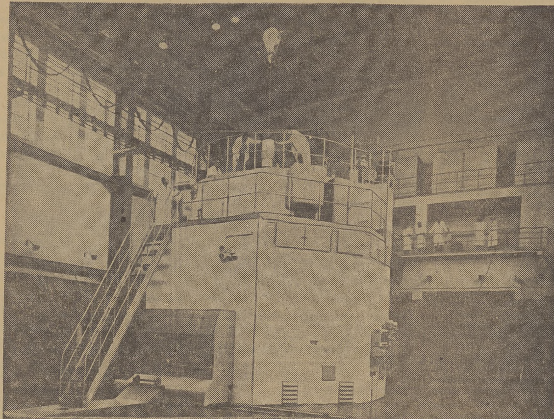
В Венгерской Народной Республике вступил в строй экспериментальный атомный реактор мощностью 2 мегаватта, построенный с помощью Советского Союза. Реактор предназначен для научно-исследовательских работ и подготовки специалистов по использованию атомной энергии в мирных целях.
