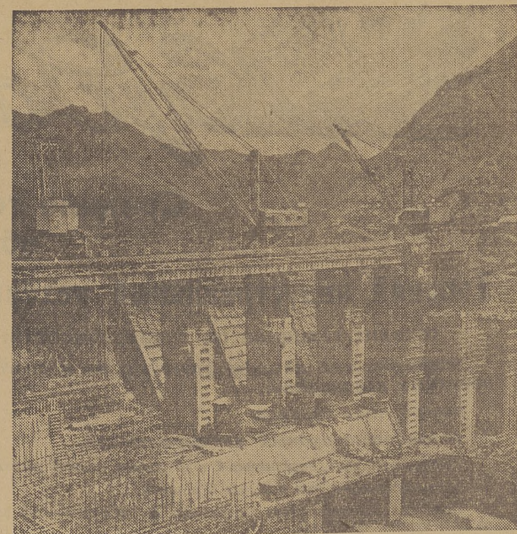
КИТАЙСКАЯ НАРОДНАЯ РЕСПУБЛИКА. В этом году даст первый ток гидроэлектростанция мощностью 580 тысяч киловатт, строящаяся в провинции Чжэцзян на реке Синьаньцзян. На снимке: строительство плотины ГЭС. (Фотохроника ТАСС).
