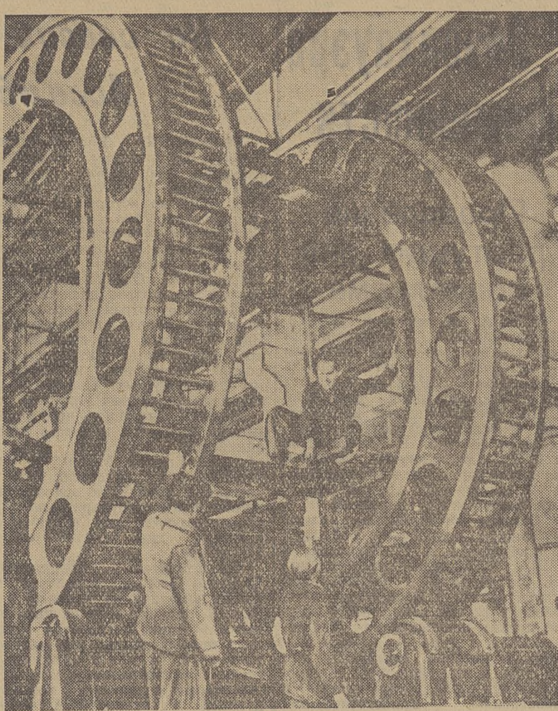
МОСКОВСКАЯ ОБЛАСТЬ. В первом механосборочном цехе Электростальского завода тяжелого машиностроения идет сборка созданной коллективом инженеров предприятия оригинальной машины, предназначенной для механизации ряда операций в литейном производстве.
