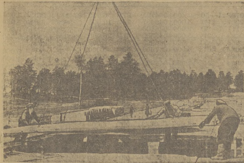
Всему миру известен молодой Ангарск — город строителей одной из величайших в мире гидростроек. Его строители применяли вместо пустотных плит перенятый technique железобетонные панели размером «на комнату» и толщиной 8 сантиметров. На снимке: укладка такой панели с помощью башенного крана.
