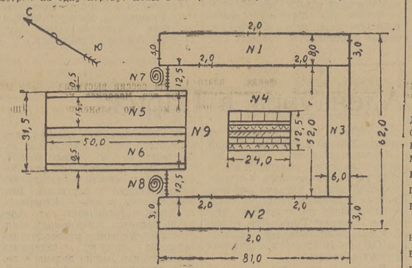
Рис. 1. План размещения фермы на 300 голов, где введено беспривязное содержание коров. 1 и 2 — коровники; 3 — извяс; 4 — доильный зал; 5, 6 — наземные силосные траншеи; 7 — стога сена; 8 — стога соломы; 9 — дворовая площадка. Верхняя стрелка С-Ю указывает северное и южное направления
