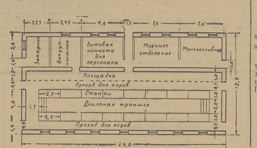
Рис. 2. План доильного зала на 16 коров.
