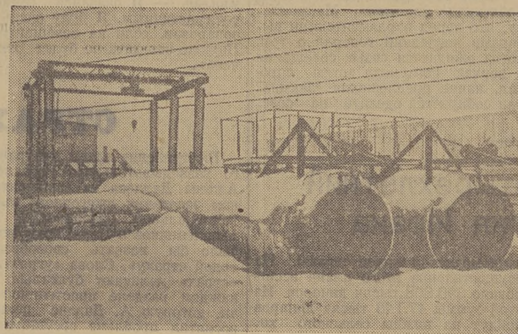
На этой установке по производству газозолотобетона можно готовить до 250 кубометров изделий в месяц. Но руководители треста «Стройдеталь» не приняли мер к ее утеплению, и установка «замерзла».
