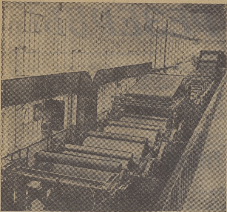
РУМЫНСКАЯ НАРОДНАЯ РЕСПУБЛИКА. На берегу Дуная близ Браилова сооружается крупный комбинат по производству целлюлозы и бумаги из камыша, в изобилии произрастающего в дельте Дуная. Строительство его ведется в сотрудничестве с ГДР, Чехословакией и Польшей. Недавно вступила в строй фабрика многослойного картона производственной мощностью 9 тысяч тонн в год. На снимке: в цехе автоматического производства картона. (Фотохроника ТАСС).
