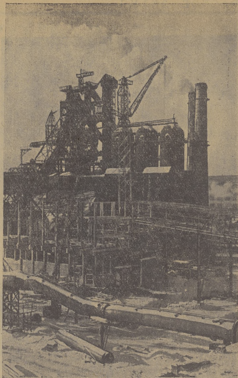
КАЗАХСКАЯ ССР. Горячие дни сейчас на строительстве Карагандинского металлургического завода в Темп-Тау. Готовится к пуску первая казахстанская домна имени 40-летия комсомола. Монтанжники выполнили огромный объем работ. Они ежедневно укладывали около 800 кубометров бетона, собирали десятки тонн металлоконструкций, много различного технологического оборудования.
