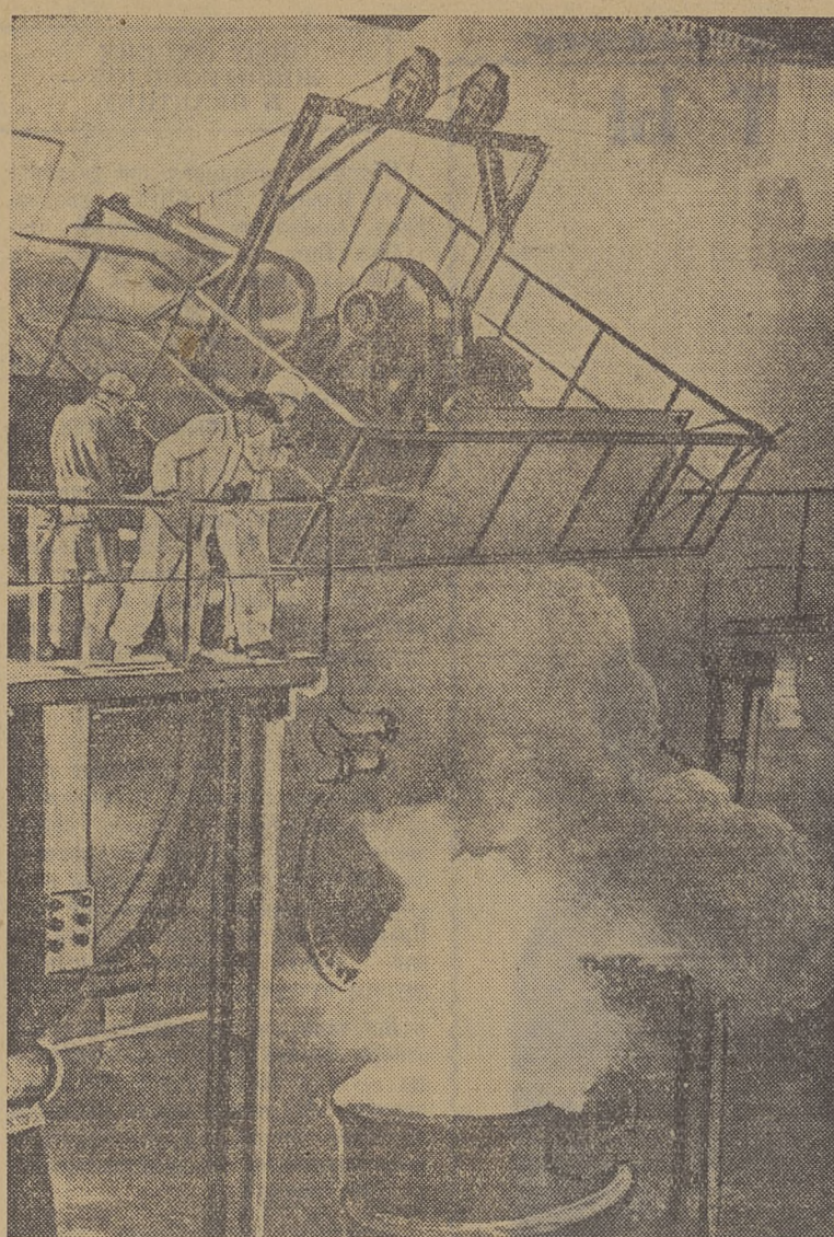
КОРЕЙСКАЯ НАРОДНО-ДЕМОКРАТИЧЕСКАЯ РЕСПУБЛИКА. Слия чугуна из миксера на металлургическом заводе имени Ким Чика (провинция Северный Хамген).
