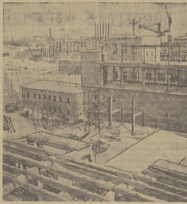
ОМСК. Рядом с нефтеперерабатывающим заводом строится завод синтетического топлива. Сырьем для нового предприятия будут служить отходы от переработки нефти. На снимке: строящийся завод синтетического топлива. (Фотохроника ТАСС).
