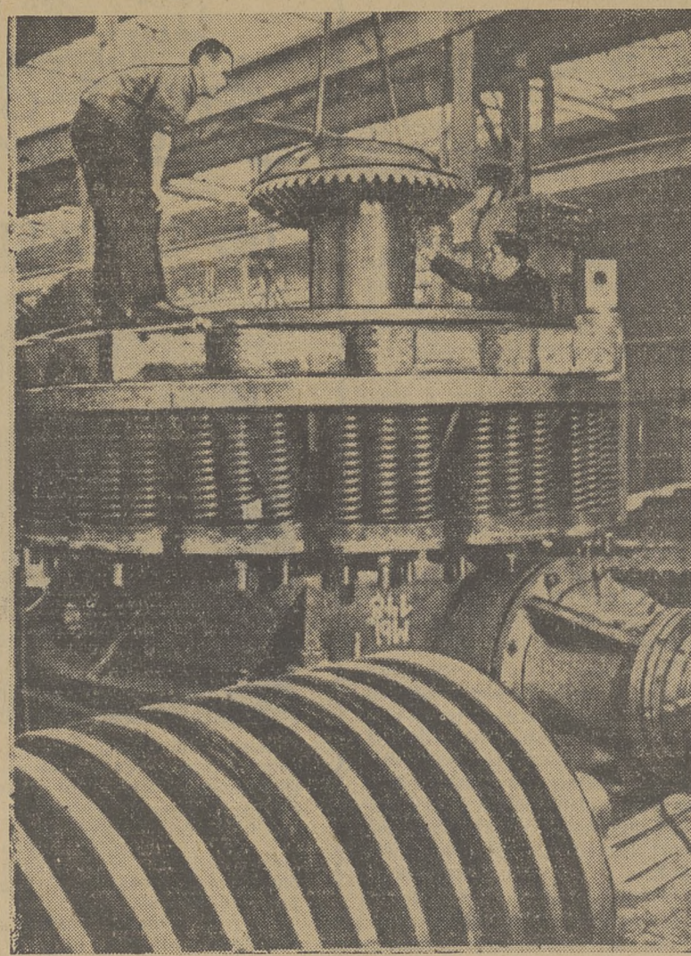
ГЕРМАНСКАЯ ДЕМОКРАТИЧЕСКАЯ РЕСПУБЛИКА. На заводе тяжелого машиностроения имени Эрнста Тельмана в Магдебурге создана крупнейшая в мире конусная дробилка. Она измельчает в течение часа до 500 кубических метров породы. Дробилка будет демонтировать на весенней Лейпцигской ярмарке.
