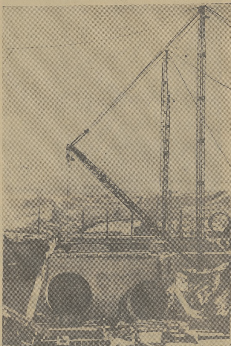
ДАГЕСТАНСКАЯ АССР. На левом берегу реки Сулак сооружается Чирюртовская ГЭС. Гидростроители обязались сдать ее в эксплуатацию на год раньше намеченного срока. Слово у них не расходуется с делом. Все основные работы ведутся с опережением графика. На снимке: строительство станционного узла.
