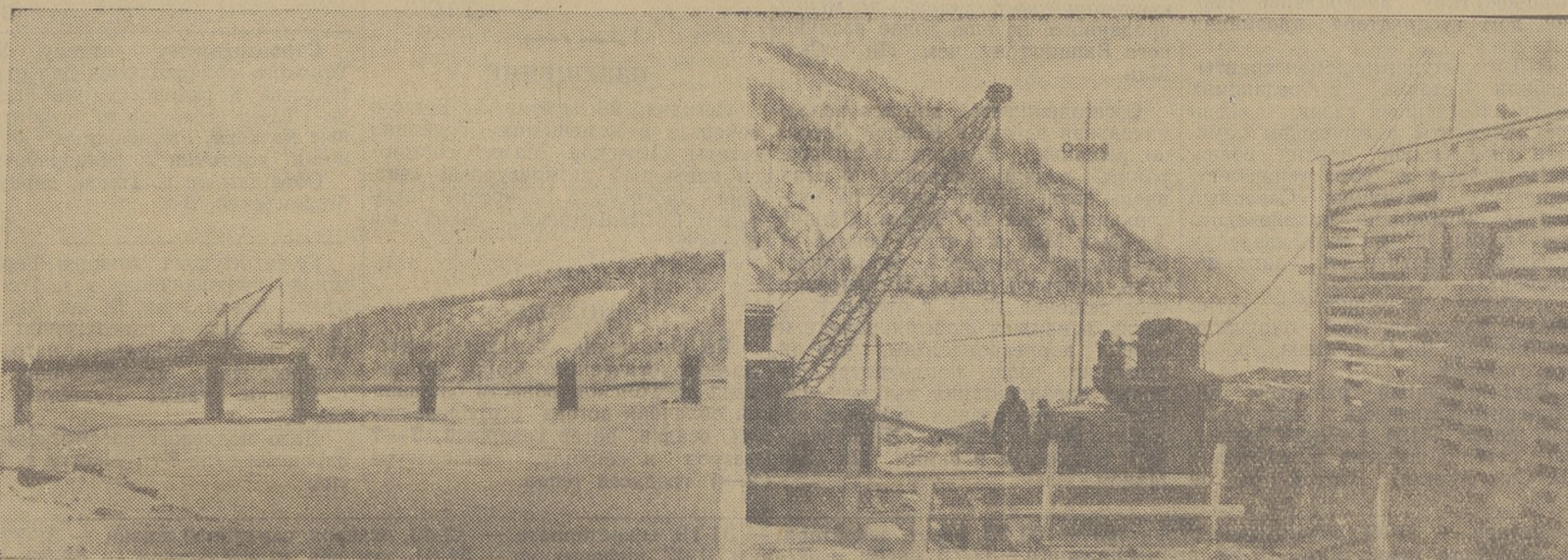
Сегодня на строительстве Красноярской ГЭС. Скоро большой мост (на снимке слева) свяжет оба берега великой стройки. Справа — пройдет еще несколько часов, и кессон будет опущен на дно Енисея. Фото И. Кузьменко.
