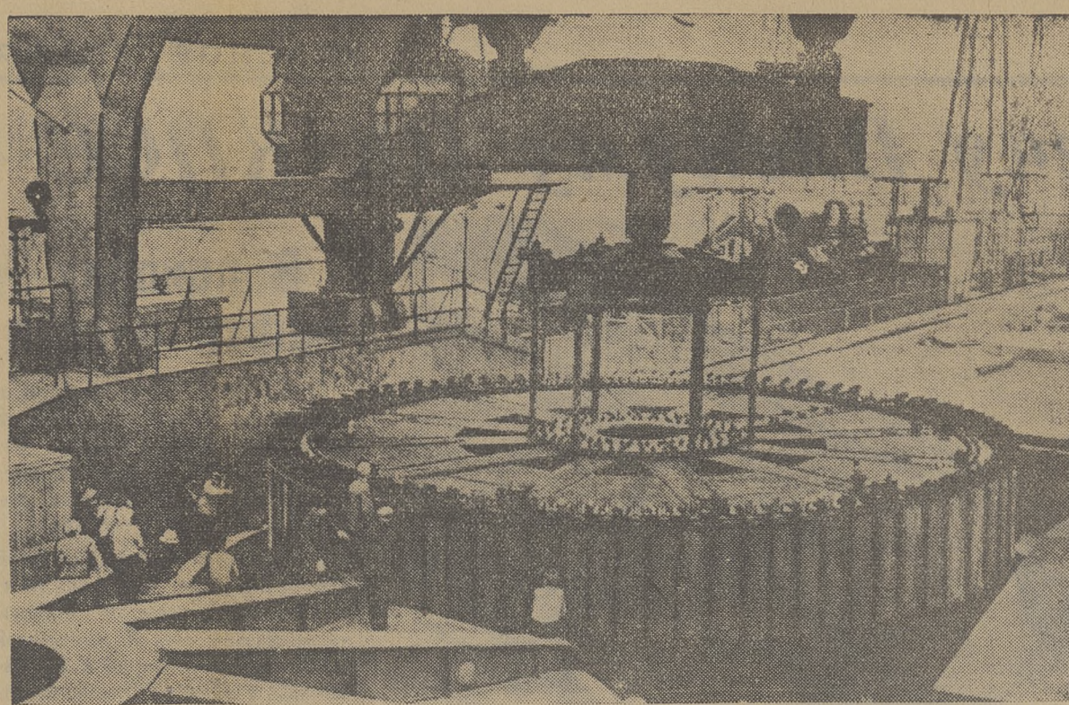
УКРАИНСКАЯ ССР. Строители Кременчугской ГЭС заложили обязательство — к 43-й годовщине Ве- ликого Октября ввести в действие все 12 гидроагре- гатов электростанции. Недавно, почти на месяц рань- ше срока, предусмотренного обязательством, был сдан в эксплуатацию седьмой гидроагрегат. Теперь быстрыми темпами ведется монтаж восьмого и девя- того агрегатов станции.
