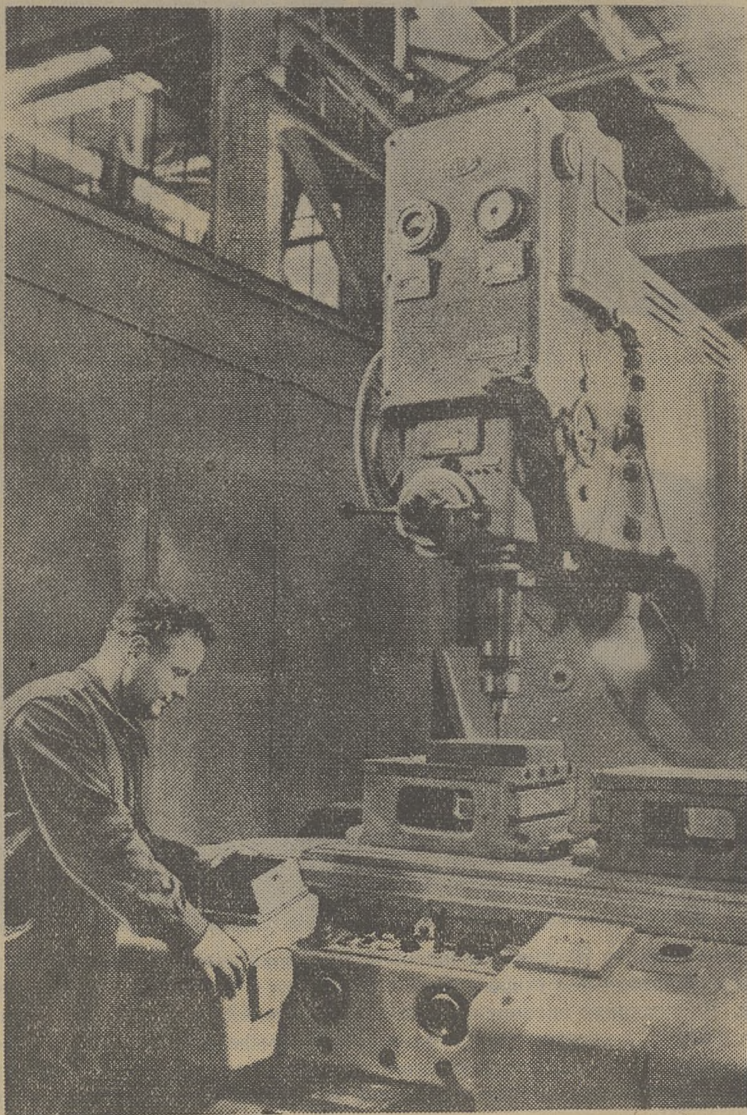
МОСКВА. Коллектив завода координатно-расточных станков создал первый в Советском Союзе координатно-расточный станок с программным управлением. Новый станок обладает точностью до 4 микронов. Он предназначен для инструментальной промышленности. Первый такой станок успешно прошел заводские испытания. На снимке: расточник Н. В. Лихачев испытывает новый станок. (Фотохроника ТАСС).
