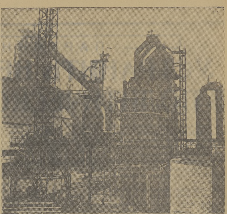
КРИВОЙ РОГ. На металлургическом заводе имени Ленина завершены работы по сооружению новой доменной печи. Эта печь — первая из серии сверхмощных чушноплавильных агрегатов, принятых на вооружение металлургической промышленности СССР в семилетке. На снимке: новая кривоножская доменная печь. (Фотохроника ТАСС).
