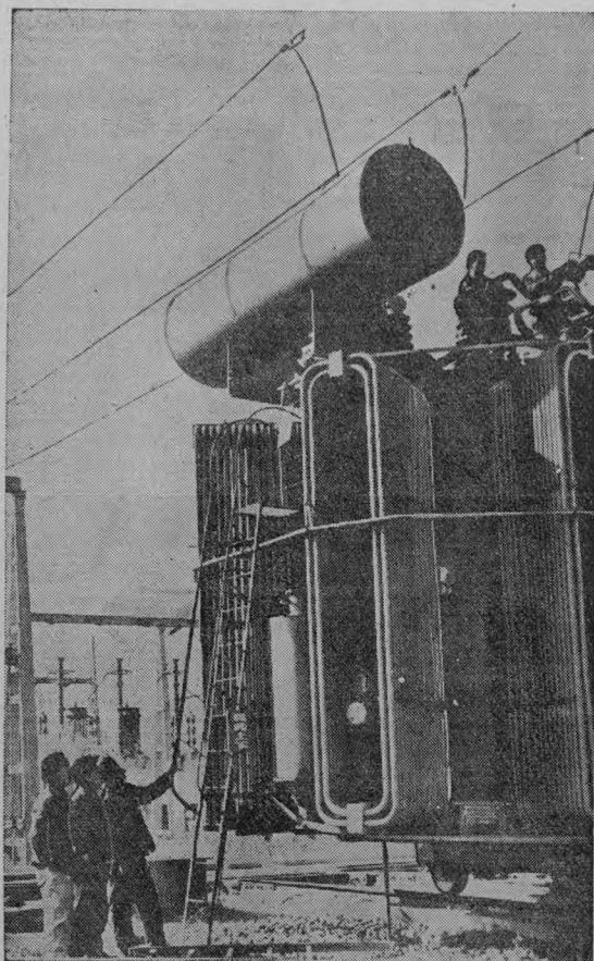
КИТАЙСКАЯ НАРОДНАЯ РЕСПУБЛИКА. Монтаж трансформатора на электростанции обогатительной фабрики на железнодорожном месторождении Дае (Центральный Китай). (Фотохроника ТАСС).
