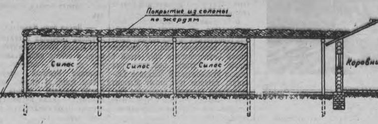
Схема закладки наземных буртов силоса у коровников (рис. 2)
