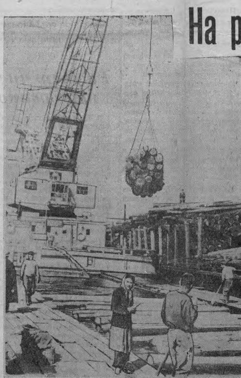
Многотонные пучки леса укладывает кран ПК-10 на палубы барж.
