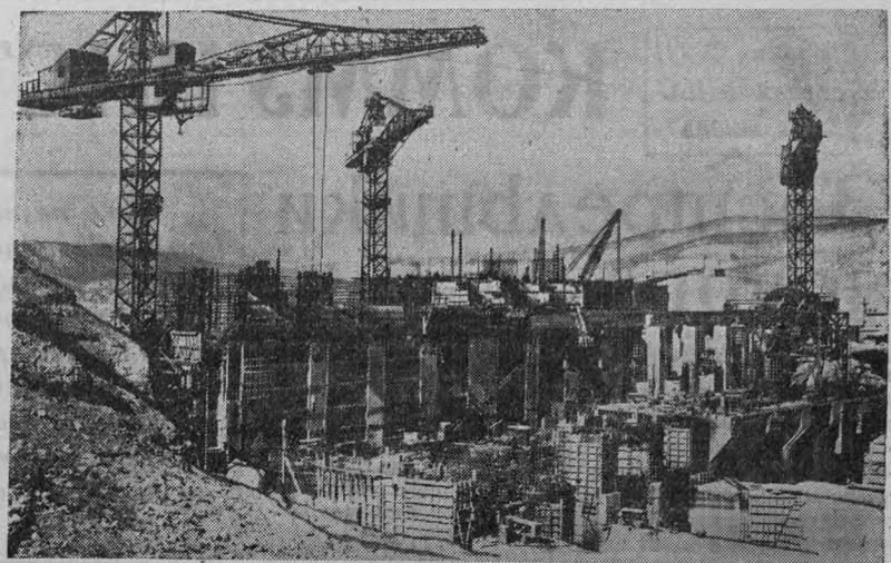
На границе Узбекистана и Киргизии завершается строительство Учкурганской ГЭС. Плотина Учкурганской ГЭС
