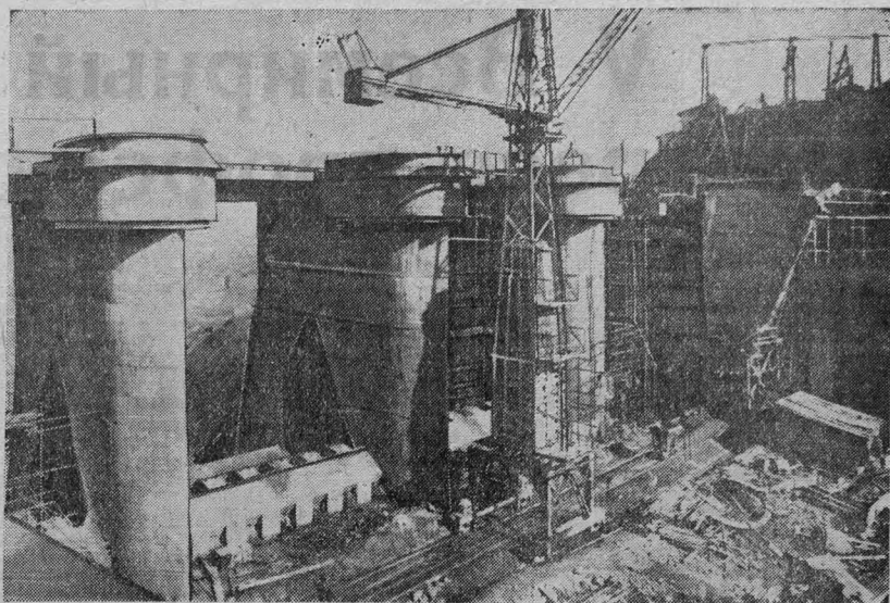
НАРОДНАЯ РЕСПУБЛИКА БОЛГАРИЯ. На реке Арде — одной из самых полноводных рек страны — будет сооружено шесть крупных и несколько мелких водохранилищ, воды которых приведут в движение турбины мощных электростанций. Водохранилище и электростанция «Студен-Кладен» уже построены и эксплуатируются. В этом году вступит в строй водохранилище «Кырджали».
