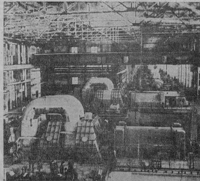
ЧЕЛЯБИНСКАЯ ОБЛАСТЬ. На Южноуральской ГРЭС готовится к сдаче новый энергоблок. С вводом в эксплуатацию турбогенератора мощностью в 200 тысяч киловатт Южноуральская ГРЭС достигнет мощности в один миллион киловатт и станет самой крупной тепловой электростанцией на Урале.
