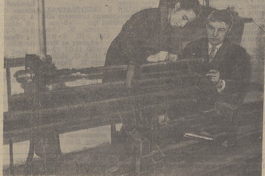
На снимке: руководитель лаборатории Г. Д. Полосаткин и аспирантка Н. Ф. Дроздова за подготовкой очередного опыта по сверхскоростному резанию металлов.
