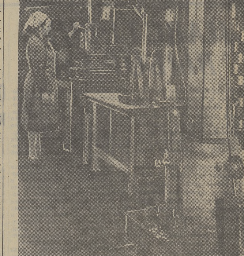
В цехе железнодорожных подшипников на Томском подшипниковом заводе все кольца подшипников после термической обработки проходят специальную проверку. Для того, чтобы обнаружить брак, на заводе изготовлены магнитный дефектоскоп и пропускная ванна с подсыпником. Применение их позволило значительно повысить качество железнодорожных подшипников.
