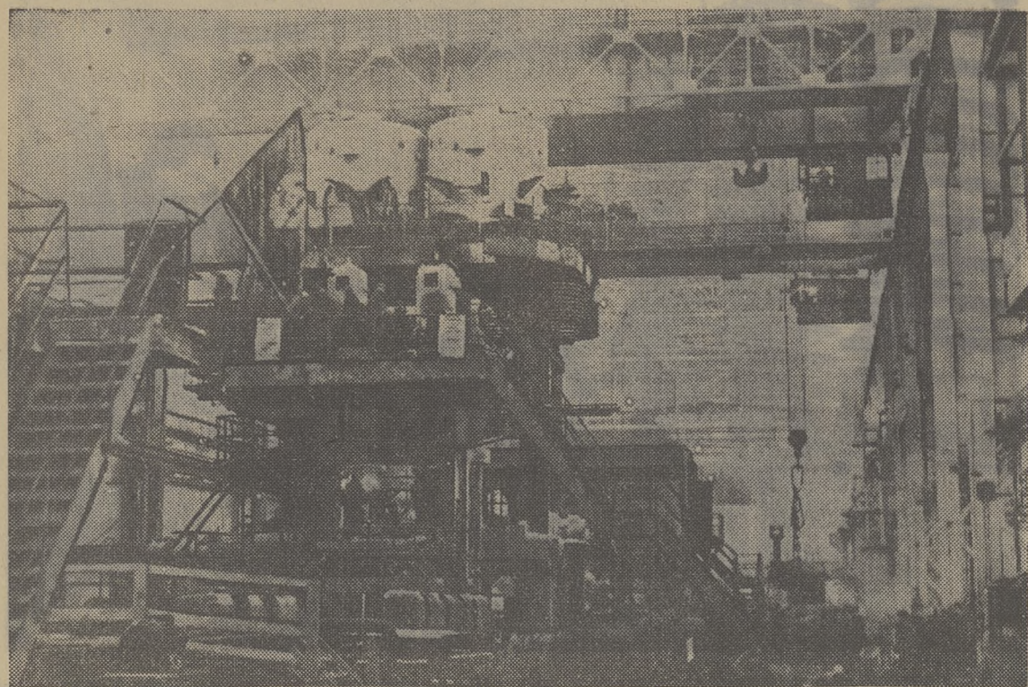
ДОНЕЦКАЯ ОБЛАСТЬ. Заканчиваются последние приготовления к пуску слябига «1150», построенного на Ждановском металлургическом заводе имени Ильича. Сель с половинной тонны оборудования, смонтированного на железобетонных основаниях, составили поточную линию, в которую входят десятки машин и механизмов. Самая крупная из них — рабочая клеть. В ее валках будут прокатываться 28-тонные стальные слитки. По техническому совершенству новый слябиг не имеет себе равных в стране.
