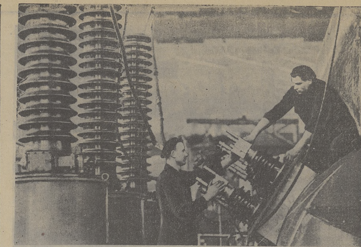
На Запорожском трансформаторном заводе в канун нового года была закончена сборка шестого мощного трансформатора для Братской ГЭС. В настоящее время он подготавливается к испытаниям.
