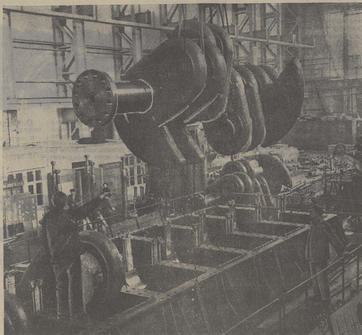
Брянский машиностроительный завод должен в этом году изготовить для торгового морского флота малооборотные дизели мощностью девять и пять тысяч лошадиных сил. На снимке: укладка секции коленчатого вала весом 47 тонн в фундамент рамы дизеля мощностью 9 тысяч лошадиных сил. (Фотохроника ТАСС).
