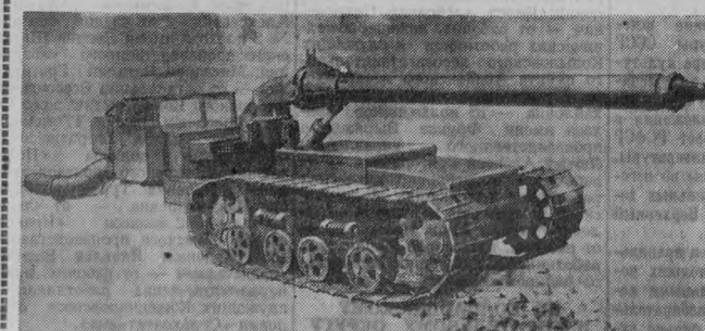
Эта «мирная пушка», созданная советскими конструкторами, надежный помощник горняков при работе в открытых карьерах.
