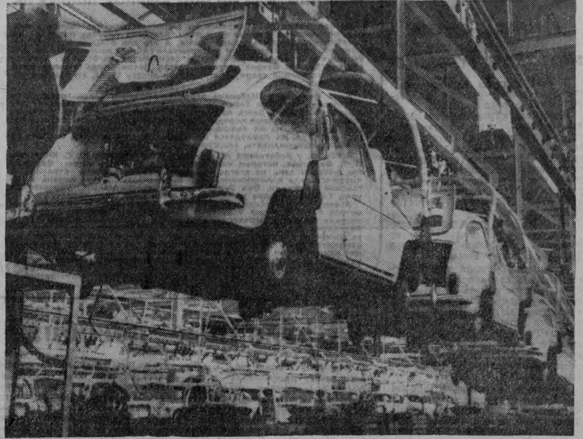
Социалистическая Федеративная Республика Югославия. Недалеко от Белграда в Крагуевце находится крупнейший автомобильный завод «Црвена Застава» («Красное Знамя»). Мощность завода 40.000 легковых и полугрузовых автомашин. В последующие годы предприятие будет выпускать до 100.000 машин в год. На снимке: в сборочном цехе завода «Црвена Застава». Фото ТАСС—ТАСС.
