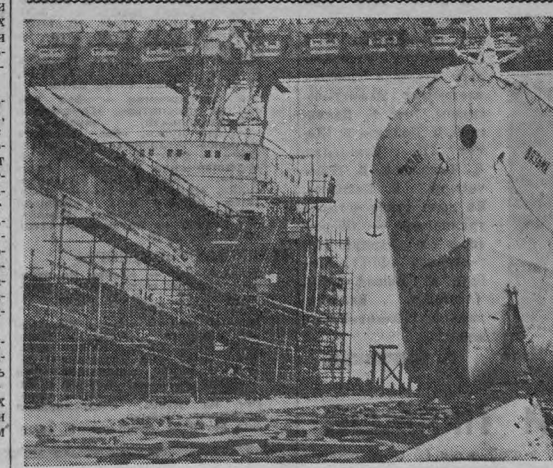
ГЕРМАНСКАЯ ДЕМОКРАТИЧЕСКАЯ РЕСПУБЛИКА. Недавно со стапелей ростоков судостроительского завода «Варновверфт» было спущено торговое судно «Вязьма» водоизмещением 12.000 тонн. Это второе из серии судов — длиной 150 метров, мощностью свыше 8.000 лошадиных сил, строящихся здесь для Советского Союза.
