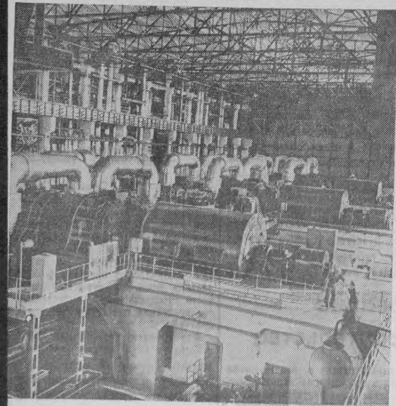
На Нововоронежской АЭС недавно пущен первый блок, электрическая мощность которого 210 тысяч киловатт. Для тепловой станции такой мощности потребовалось бы более двух тысяч тонн угля в сутки, а для первого блока АЭС — всего около 500 граммов урана-235. Начало строительства второго блока мощностью 365 тысяч киловатт. НА СНИМКЕ: общий вид машинного зала. (Фотохроника ТАСС).
