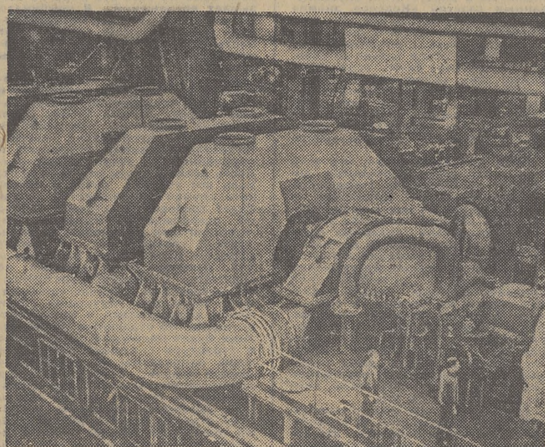
ЛЕНИНГРАД. На Металлическом заводе имени ХХII съезда КПСС изготовлена крупнейшая в Европе паровая турбина мощностью 800 тысяч киловатт.
