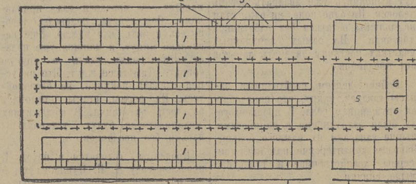
СЛЕВА — СХЕМА РАСПОЛОЖЕНИЯ ОБОРУДОВАНИЯ В КОРМУХЕ: 1 — пастоприготовитель ПЗГ-2, 2 — транс- портёр СТ-2, 3 — регулятор РМ-250 с элек- тродвигателем мощностью 2,8 квт, 4 — за- парник-смеситель-раздатчик, 5 — ком- прессор, 6 — патрубок с вентилем для вы- пуска пара, 7 — загруженный люк, 8 — за- движка-дудло, 9 — подводящая пара из термо- изоля, 10 — шланг гофрированный диаметром 100 мм.
