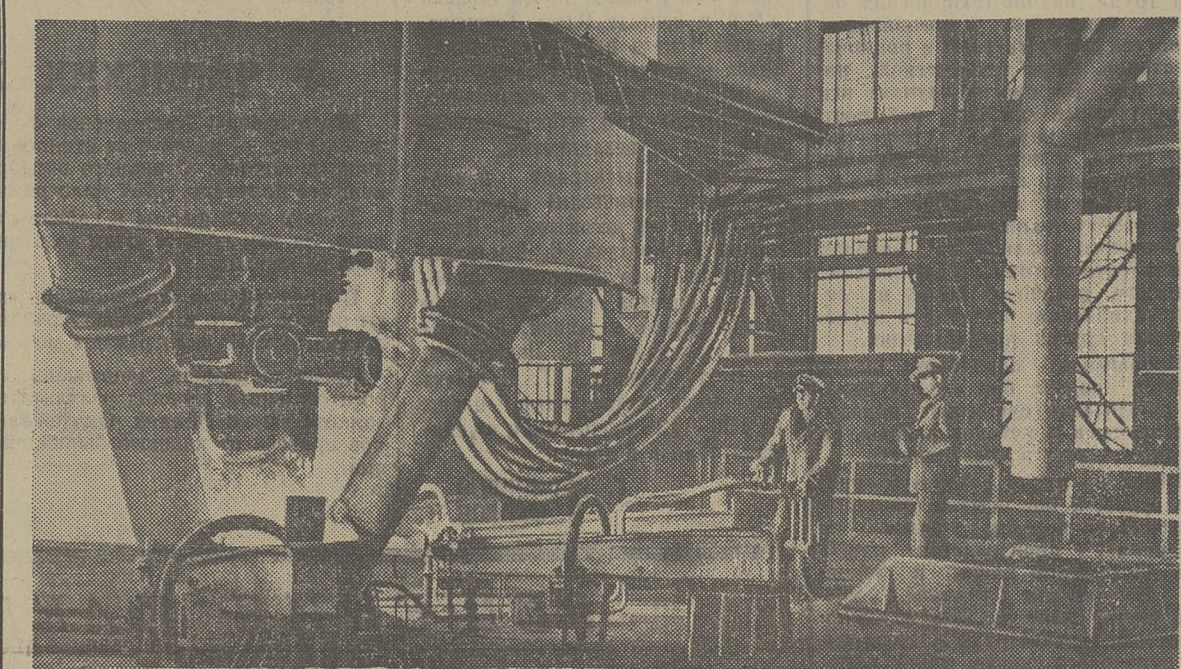
НА ЗАПОРОЖСКОМ ФЕРРОСПЛАВНОМ ЗАВОДЕ НЕДАВНО ВСТУПИЛА В СТРОЙ НОВАЯ ПЕЧЬ ЗАКРЫТОГО ТИПА. ВСЕ ПРОЦЕССЫ НА НЕЙ МЕХАНИЗИРОВАНЫ И АВТОМАТИЗИРОВАНЫ. СООРУЖАЮТСЯ ЕЩЕ ДВЕ ТАКИЕ ПЕЧИ. (Фотохроника ТАСС).
