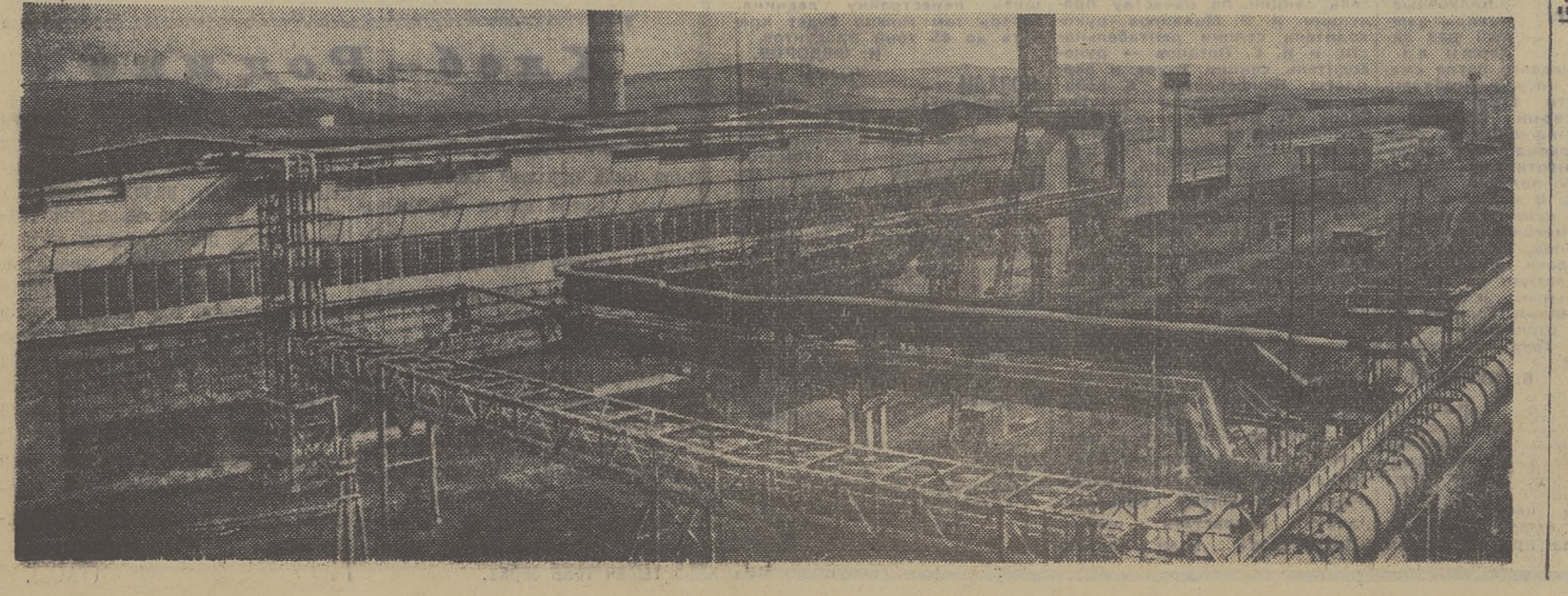
НОВОКУЗНЕЦК. Клетки мелкосортного стана «250», сооруженного на Западно-Сибирском металлургическом заводе, приняли первый металл. Идет горячее опробование — генеральная предпусковая репетиция.
