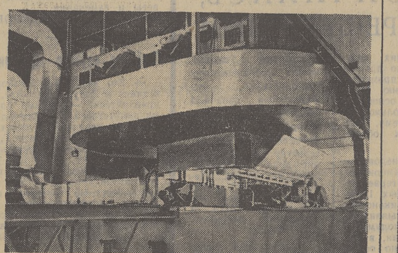
ДУБНА (Московская область). В Объединенном институте ядерных исследований создана новая экспериментальная установка для исследований в области физики элементарных частиц — двухметровая проволочная камера. По линейным размерам, определяющим длину пробега элементарных частиц, новая камера превосходит все аналогичные, имеющиеся в передовых лабораториях мира. Благодаря этому новая установка даст возможность повысить точность и эффективность исследований. Двухметровая проволочная камера установлена на одном из антипротоновых каналов синхрофазотрона. Она уже дала первые серии фотоснимков следов ядерных взаимодействий. В разработке и создании камеры принимали участие советские, болгарские и немецкие специалисты. Ряд сложных заказов выполнили советские промышленные предприятия. Юстирому оптической системы осуществил оптический институт ГДР. Физики социалистических стран получили в свое распоряжение новый первоклассный прибор, расширяющий возможности исследований материи. НА СНИМКЕ: механики готовят 2-метровую проволочную камеру к эксперименту. (Фотохроника ТАСС).
