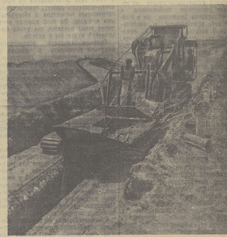
Сырдарьинская область. Сорок тысяч гектаров голодных земель спасет от засухи дренаж. Протяженность «подземных рек» уже сейчас составляет более 1.250 километров. С каждым днем трасса уходит все дальше в степь. На снимке: механизированная укладка гончарных труб горизонтального дренажа. Фото А. Горюхина. (Фотохроника ТАСС).
