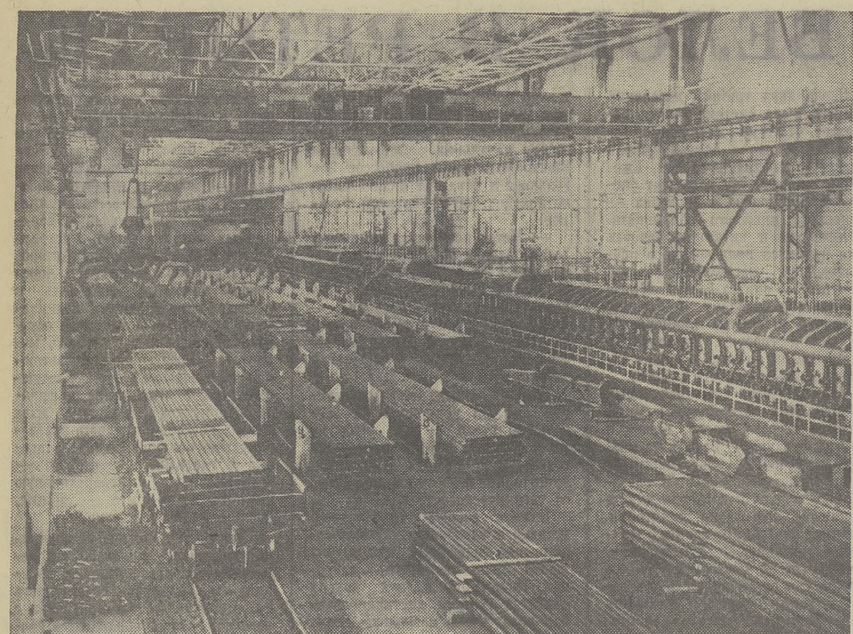
СВЕРДЛОВСКАЯ ОБЛАСТЬ. Недавно на Нижне-Тагильском металлургическом комбинате имени В. И. Ленина вступил в строй цех обменной закалки рельсов. В нем установлена автоматическая машина, позволяющая производить закалку рельсов в масле. Срок службы рельсов, обработанных таким образом, увеличивается в два раза. В течение двадцати лет они будут надежно выдерживать нагрузку, не требуя замены.
