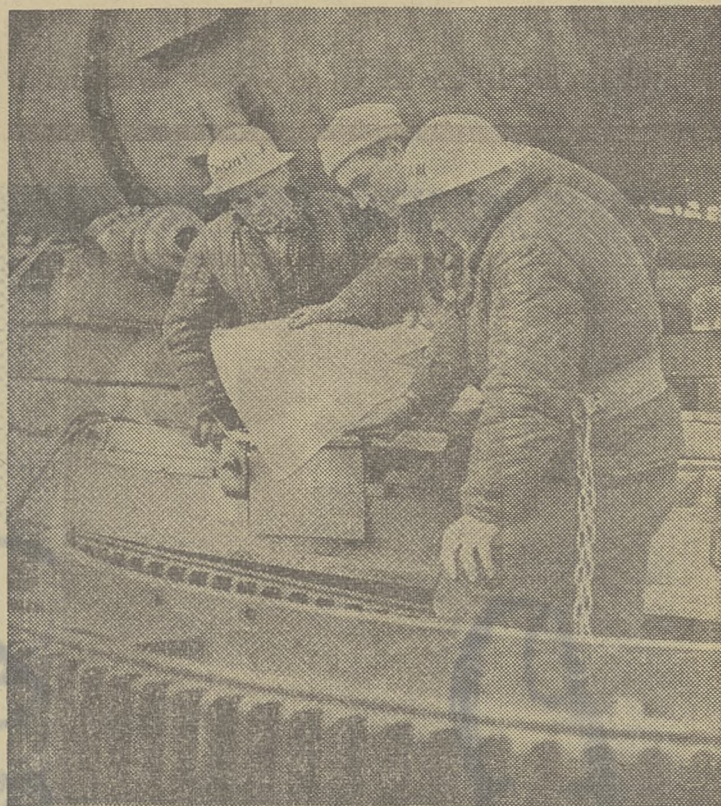
БЕЛОРУССИЯ. Недалеко от Витебска, на левом берегу реки Западной Двины, добывается доломитовый известняк, перерабатываемый заводом «Руба» в удобрения. Сейчас здесь ведется строительство еще одного завода. С вводом его в действие колхозы и совхозы страны получат еще полмиллиона тонн доломитовой муки в год.
